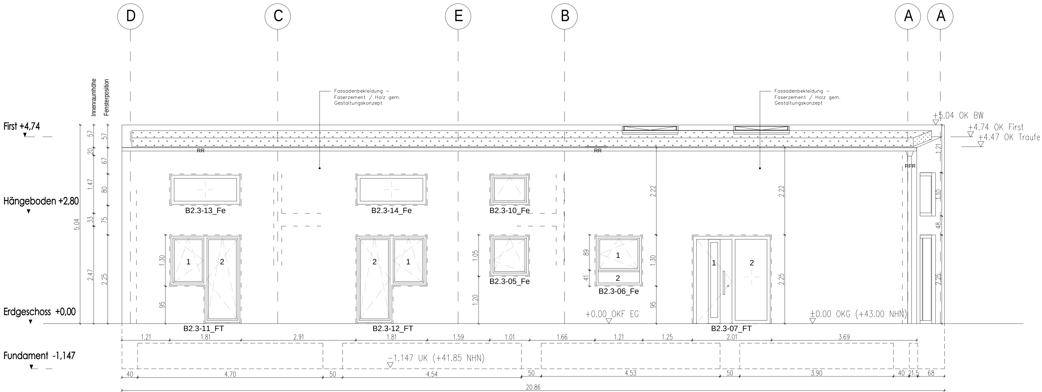
Ansicht B2.3 - Norden
