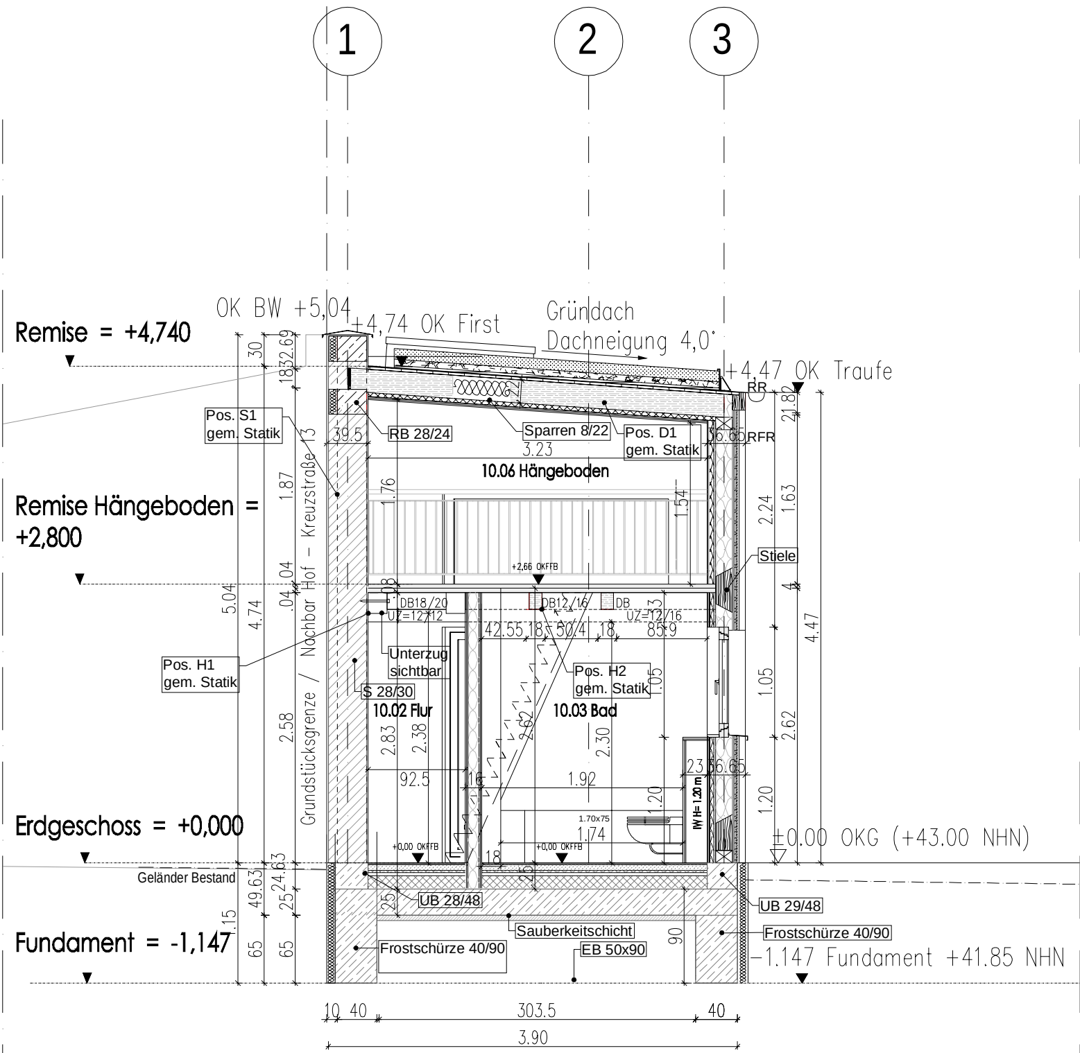
Schnitt c-c
